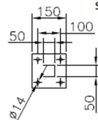
Fixation pour plan vertical ou latérale sur Mât
